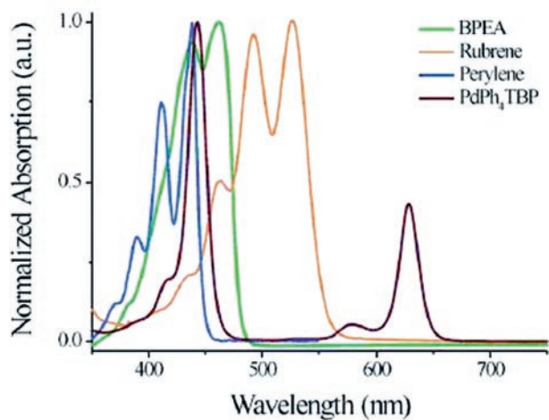
Рис. 5. Спектральные характеристики излучения органических веществ OLED
